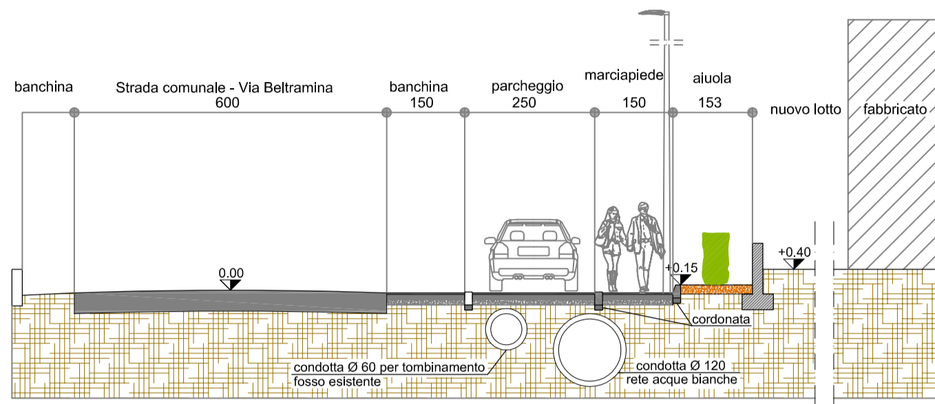
SEZIONE DI PROGETTO su Via Beltramina - scala 1:100
