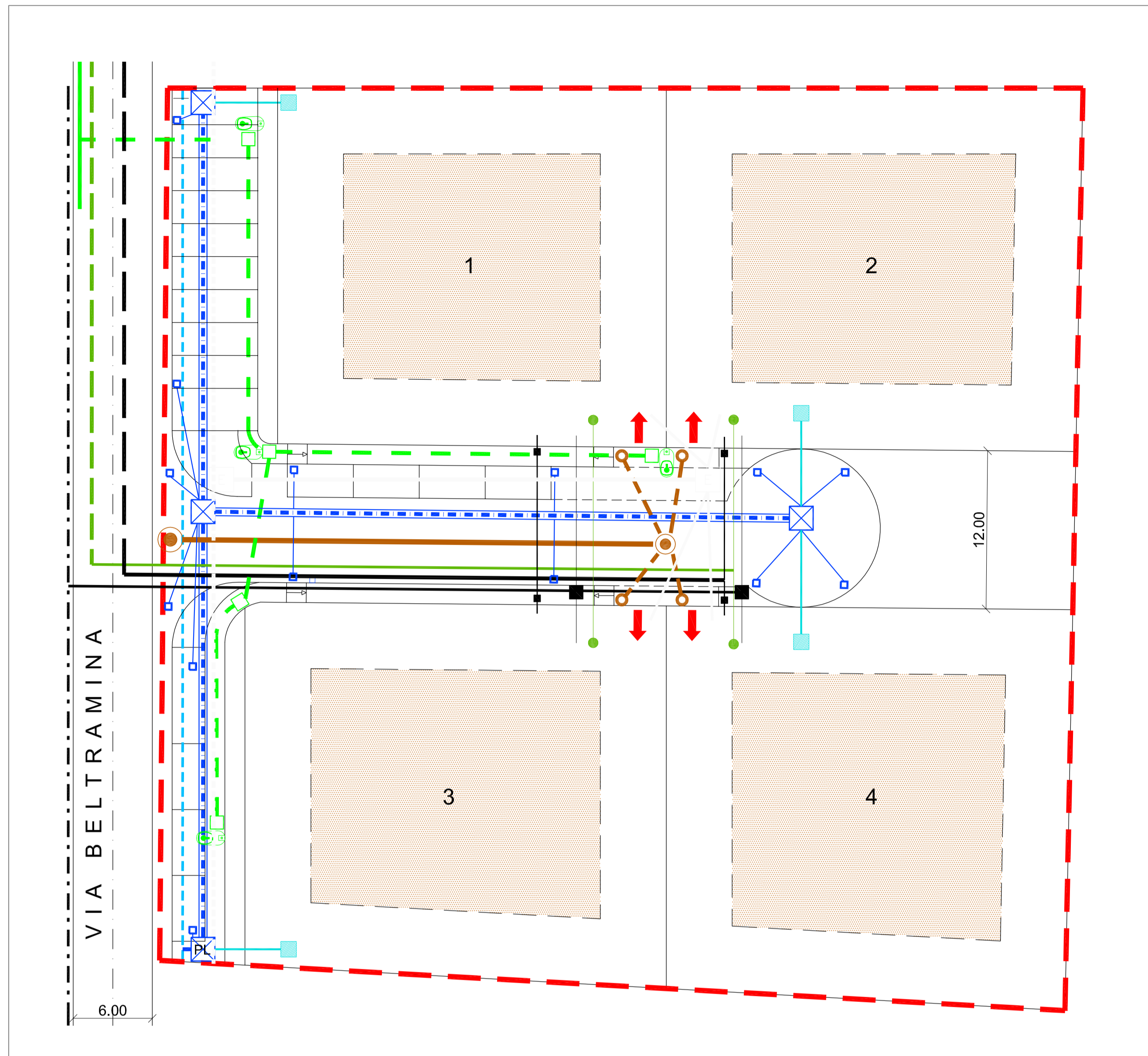
PLANIMETRIA - scala 1:250
